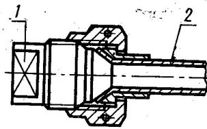
1—специальный калибр; 2—труба в сборе по ГОСТ 13954—74
