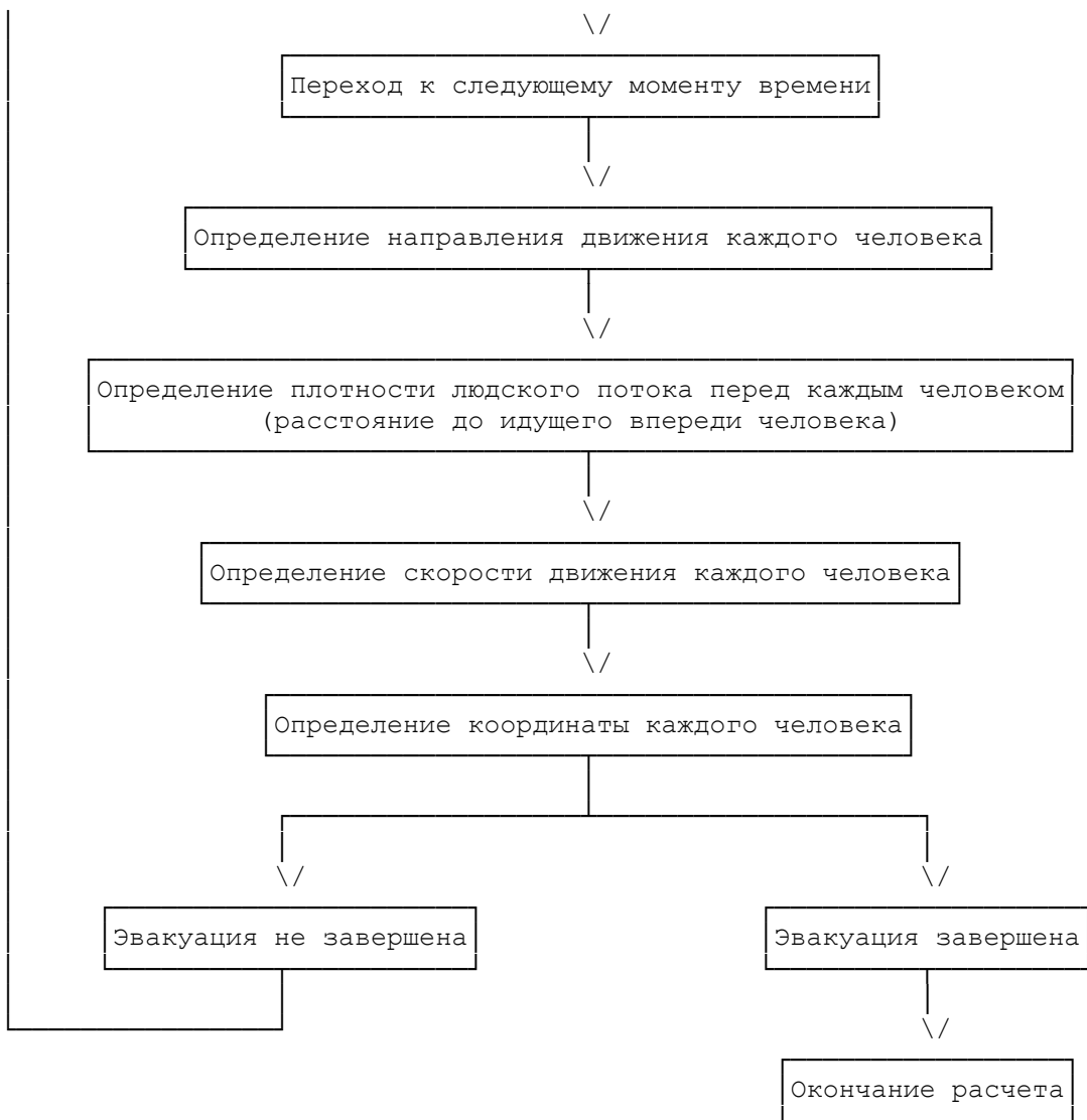
Рис. ПЗ.2. Блок-схема определения расчетного времени эвакуации людей из здания
